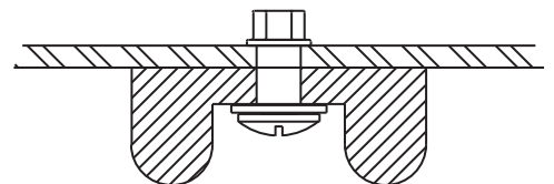
OPTIONAL RUBBER FOOT PAD
